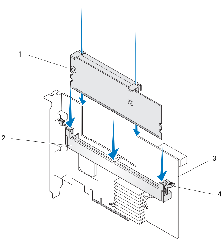
Figura 4. Instalación de un módulo de memoria dual en línea
